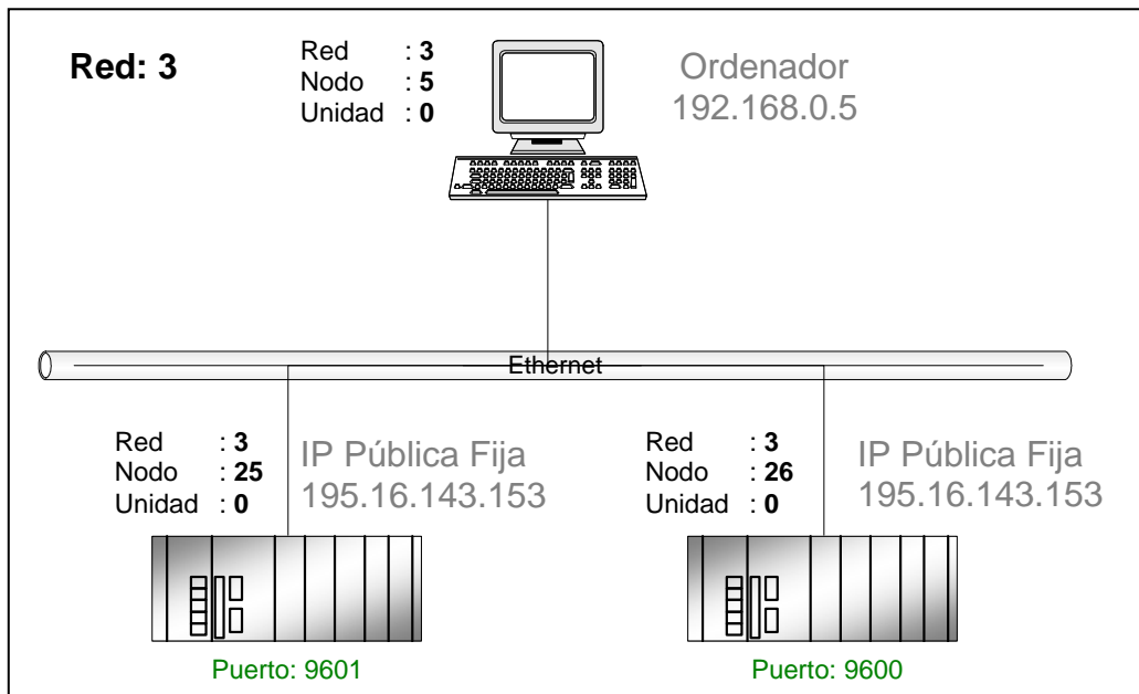
Esquema de direccionamientos FINS
